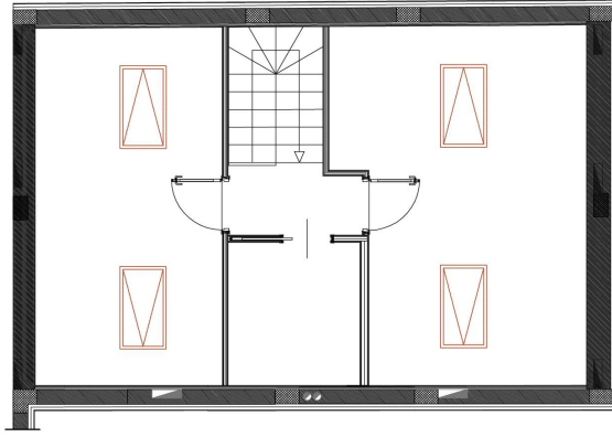
PIANTA PIANO SOTTOTETTO
